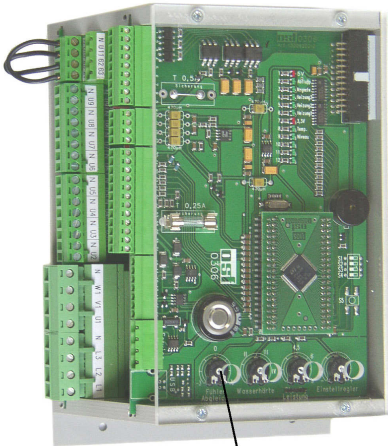
Elektronikgehäuse mit Platinen
